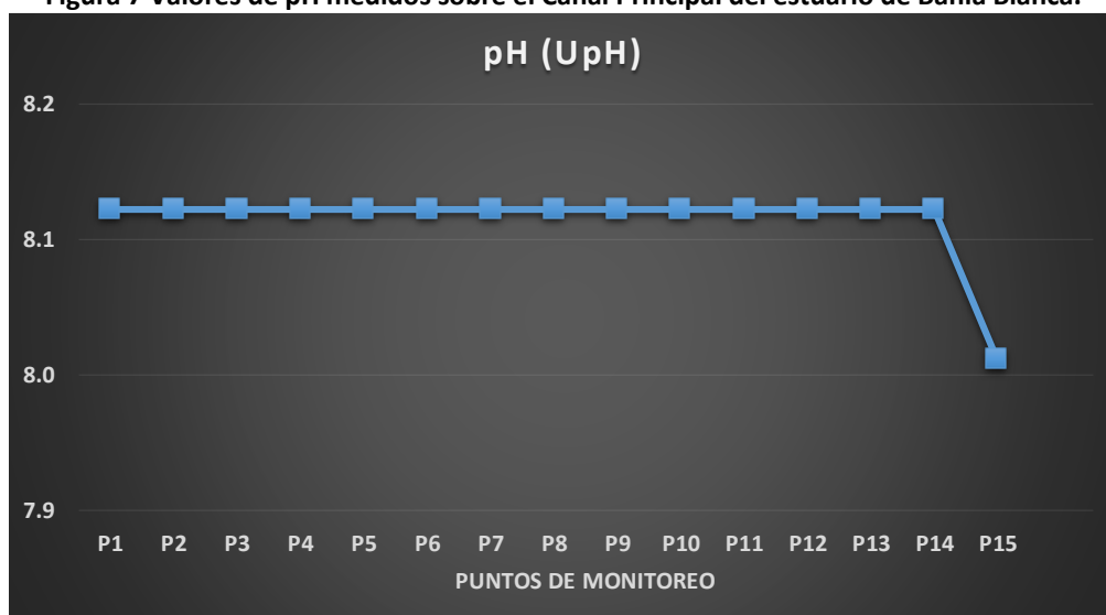
Figura 7 Valores de pH medidos sobre el Canal Principal del estuario de Bahía Blanca.
