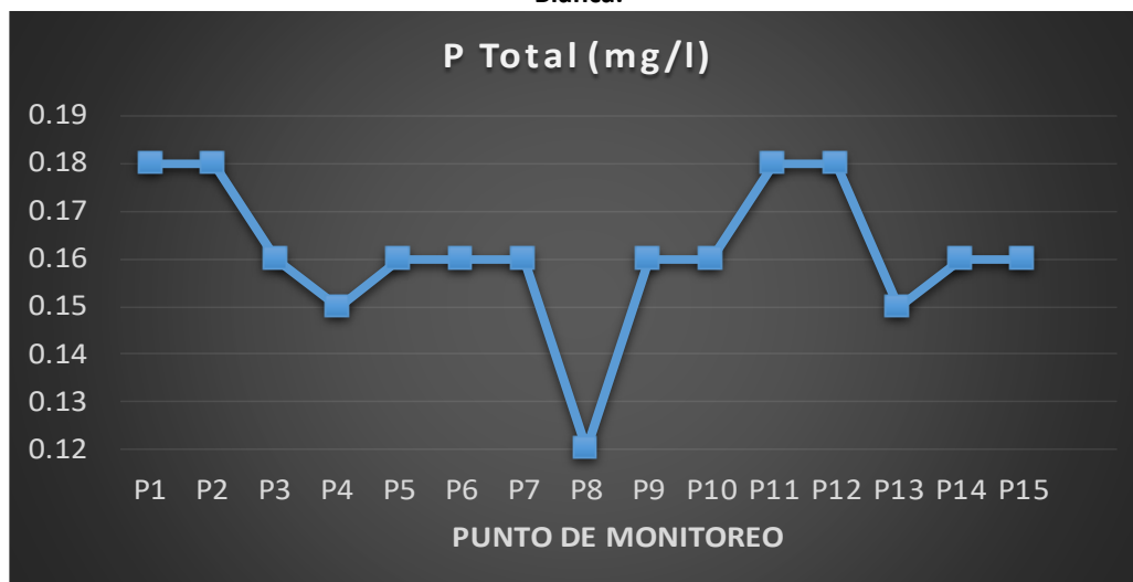
Figura 12 Valores de Fosforo Total ( P_{TOTAL} ) medidos sobre el Canal Principal del estuario de Bahía Blanca.
