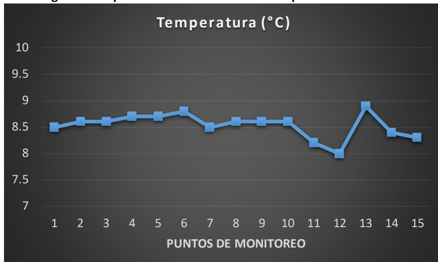
Figura 6 Temperatura medida in situ en cada punto de monitoreo.
