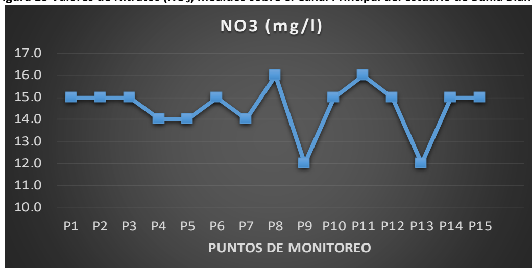
Figura 13 Valores de Nitratos ( NO_3 ) medidos sobre el Canal Principal del estuario de Bahía Blanca.
