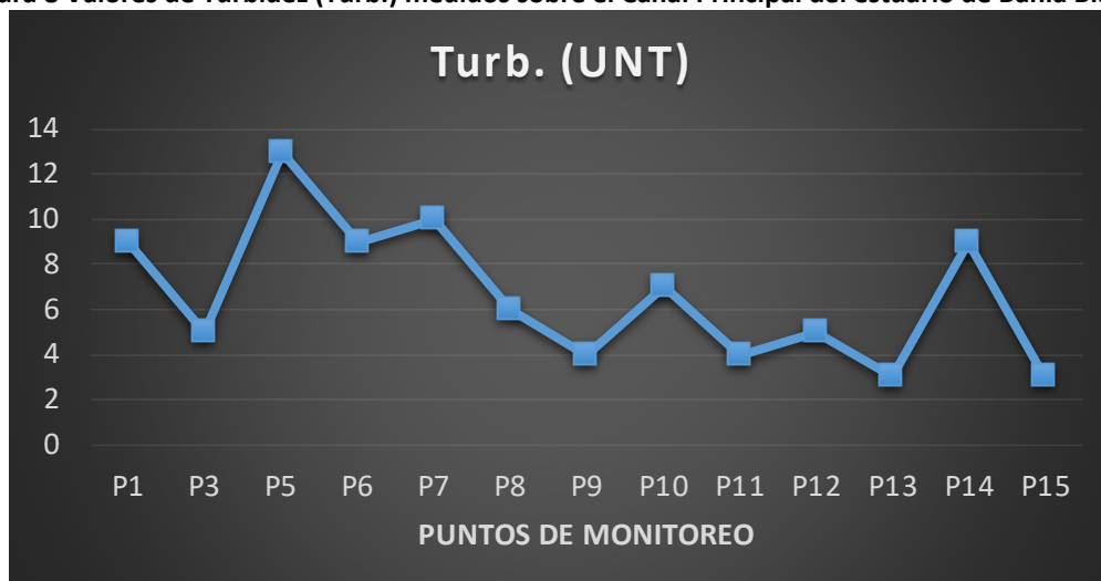
Figura 8 Valores de Turbidez (Turb.) medidos sobre el Canal Principal del estuario de Bahía Blanca.
