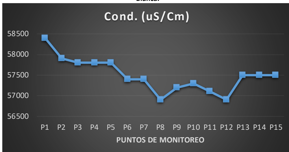
Figura 14. Valores de Conductividad (Cond.) medidos sobre el Canal Principal del estuario de Bahía Blanca.
