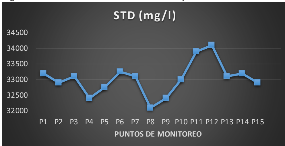
Figura 15. Valores de STD medidos sobre el Canal Principal del estuario de Bahía Blanca.
