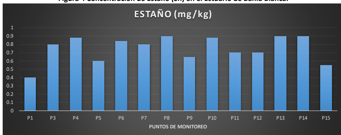
Figura 4 Concentración de Estaño (Sn) en el Estuario de Bahía Blanca.
