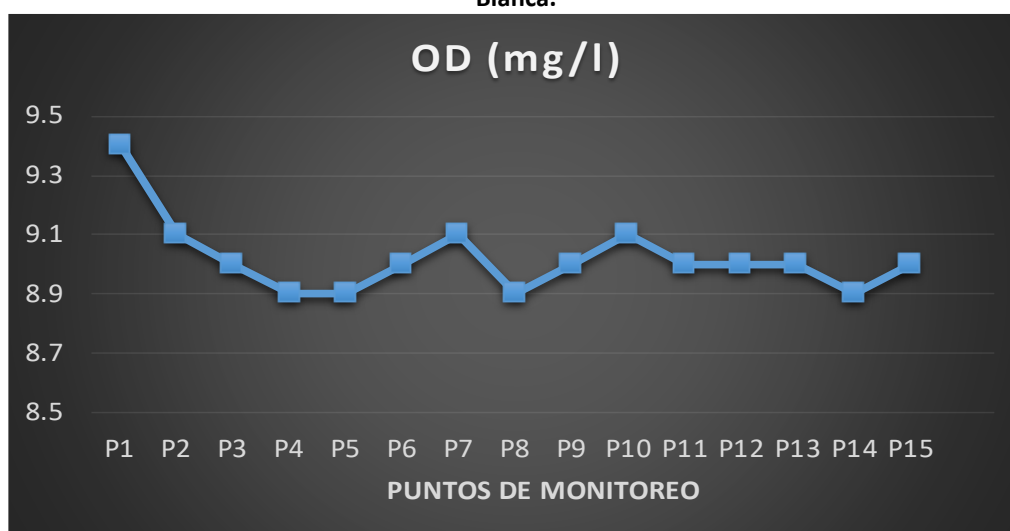
Figura 11 Valores de Oxígeno Disuelto (OD) medidos sobre el Canal Principal del estuario de Bahía Blanca.
