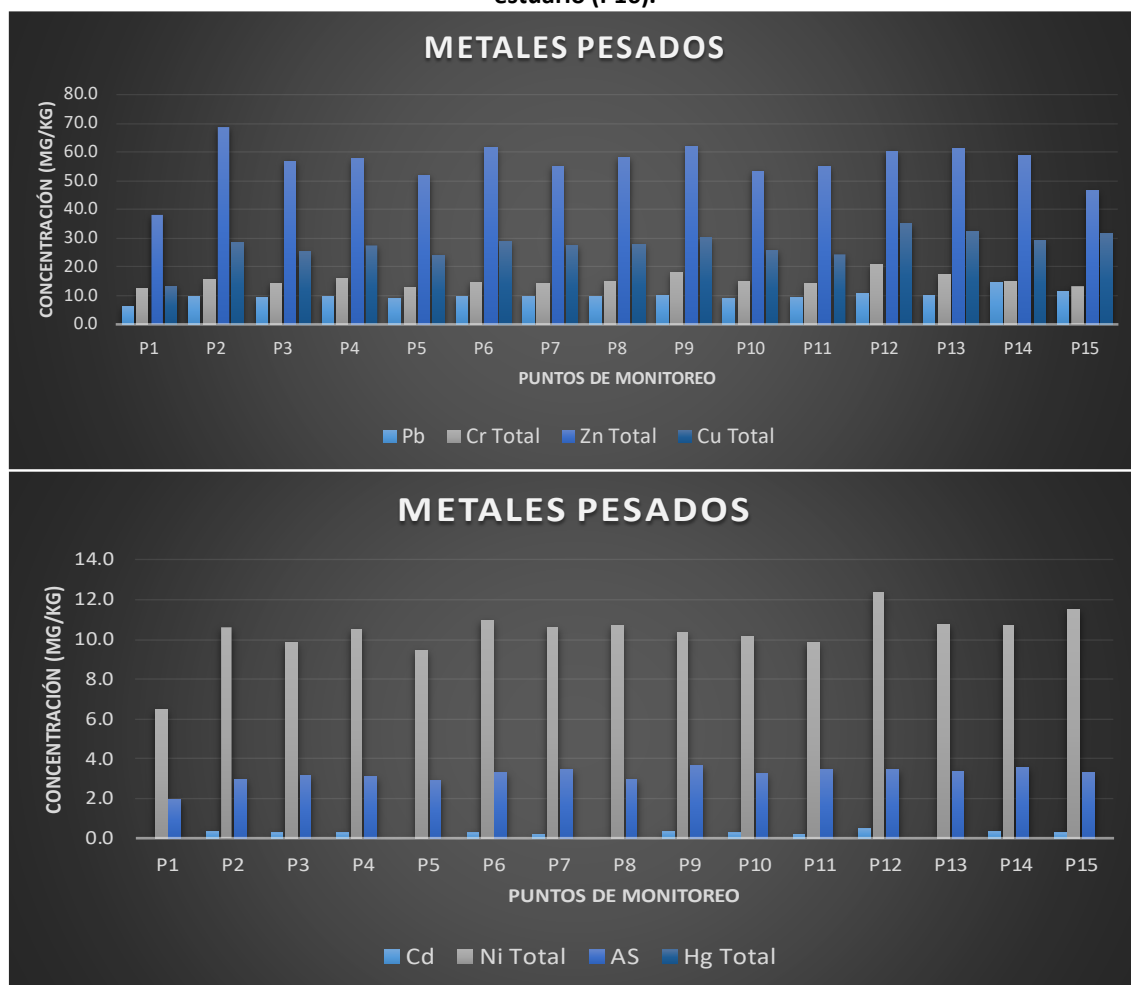
Figura 3 Concentración normalizada de metales pesados y Arsénico (mg/kg) en el estuario de Bahía Blanca. Los puntos se muestran desde el punto más externo en la boca (P1) hacia el interior del estuario (P16).
