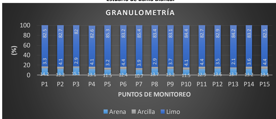
Figura 5 Análisis granulométrico en los diferentes puntos de monitoreo sobre el Canal Principal del Estuario de Bahía Blanca.
