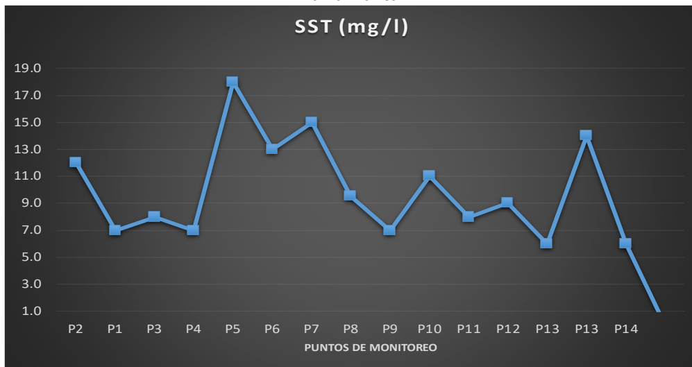
Figura 9 Valores de Solidos Suspendedos Totales (SST) medidos sobre el Canal Principal del estuario de Bahía Blanca.
