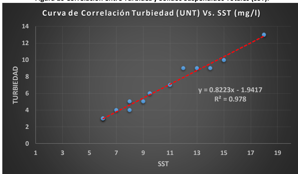
Figura 10 Correlación entre Turbidez y Solidos Suspendedos Totales (SST).
